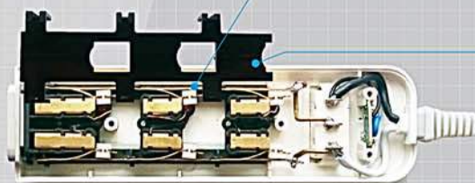
※延長線內部構造
